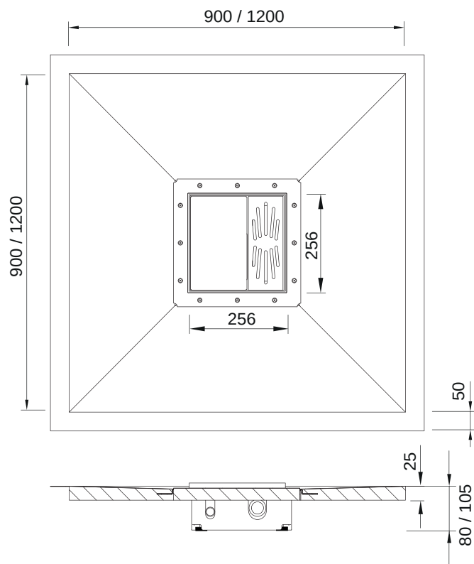
Duschbodenelement aus PUR 1200 x 1200 x 25 mm mit eingebauter Jung Plancofix Bodenablaufpumpe
