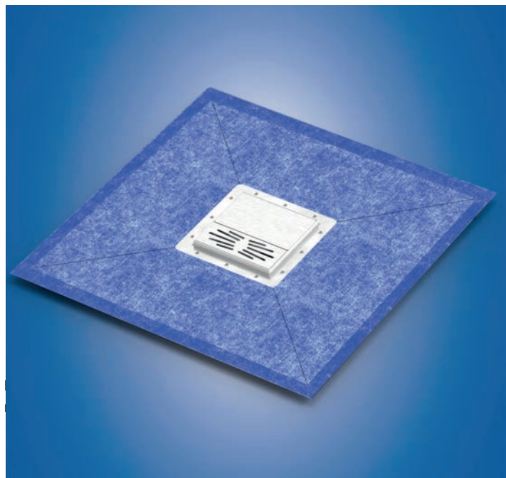
Duschbodenelement aus PUR 1200 x 1200 x 25 mm mit eingebauter Jung Plancofix Bodenablaufpumpe
